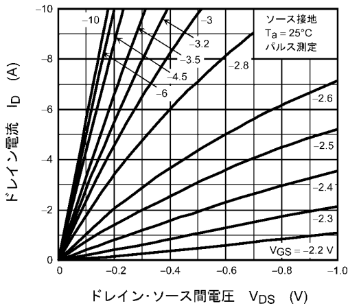
図 8.1.1 I_D - V_{DS}
