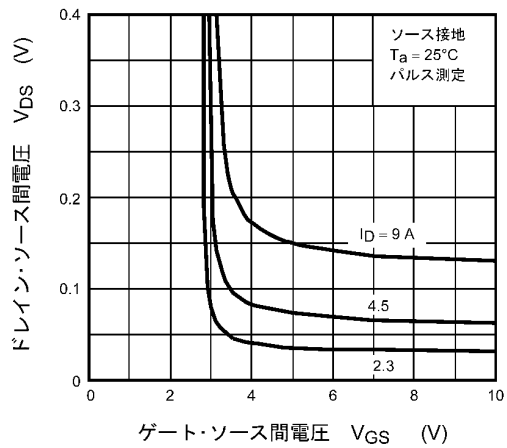
図 8.2.4 V_{DS} - V_{GS}
