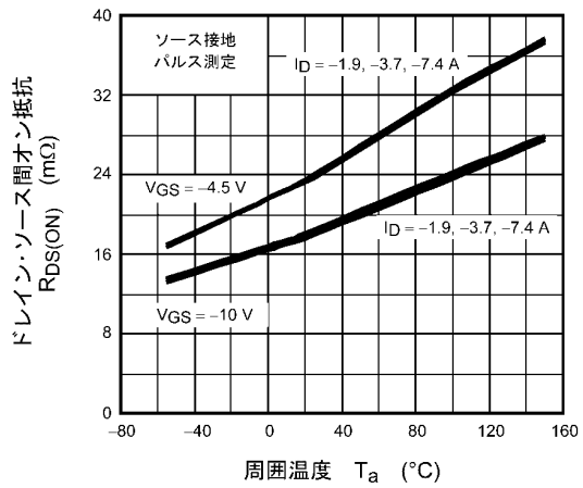
図 8.1.6 R_{DS(ON)} - T_a
