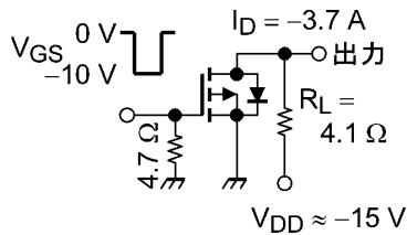
図 6.2.1 スwitchング時間の測定回路例 (P-ch)
