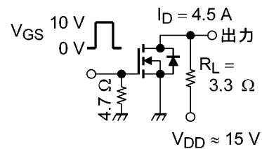
図 6.2.2 スwitchング時間の測定回路例 (N-ch)
