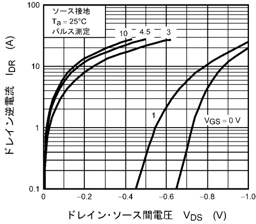
図 8.2.7 I_{DR} - V_{DS}
