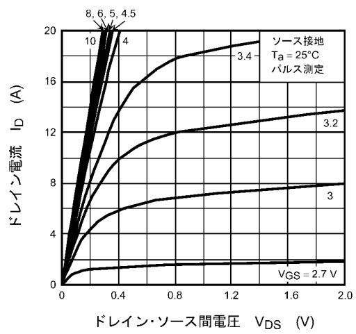
図 8.2.2 I_D - V_{DS}
