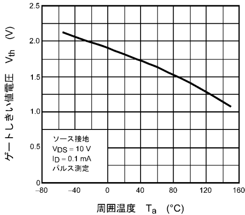
図 8.2.9 V_{th} - T_a
