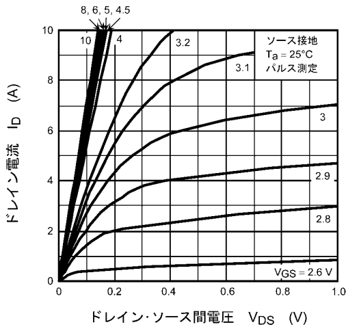
図 8.2.1 I_D - V_{DS}
