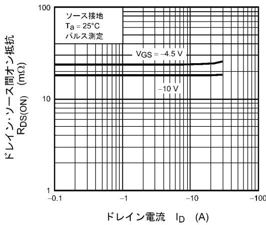
図 8.1.5 R_{DS(ON)} - I_D
