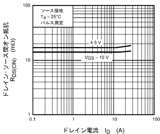
図 8.2.5 R_{DS(ON)} - I_D
