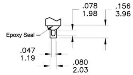
SOLDER LUG
