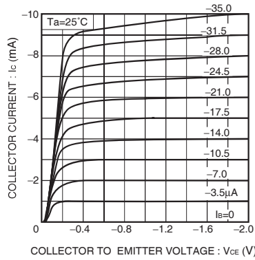
Fig.2 エミッタ接地出力静特性 (I)
