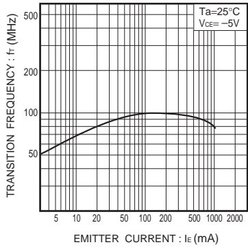
Fig.8 利得帯域幅-エミッタ電流特性
