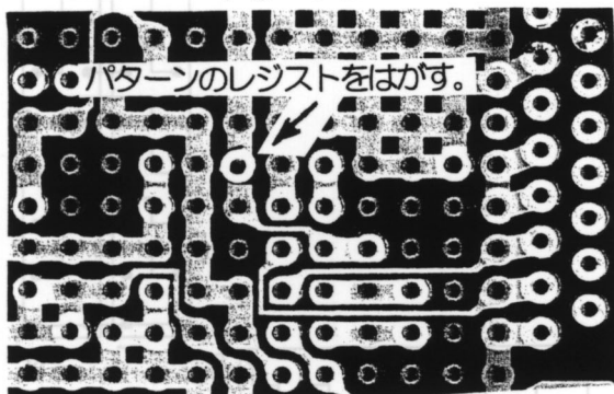
パターン面
