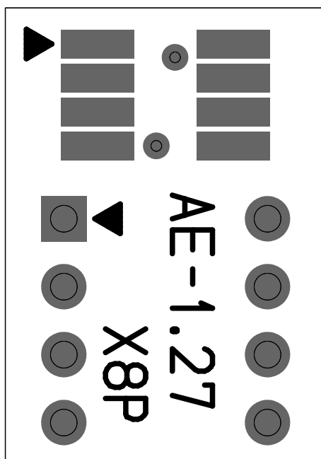
AE-1.27X8P 表面レジスト・シルク☒
