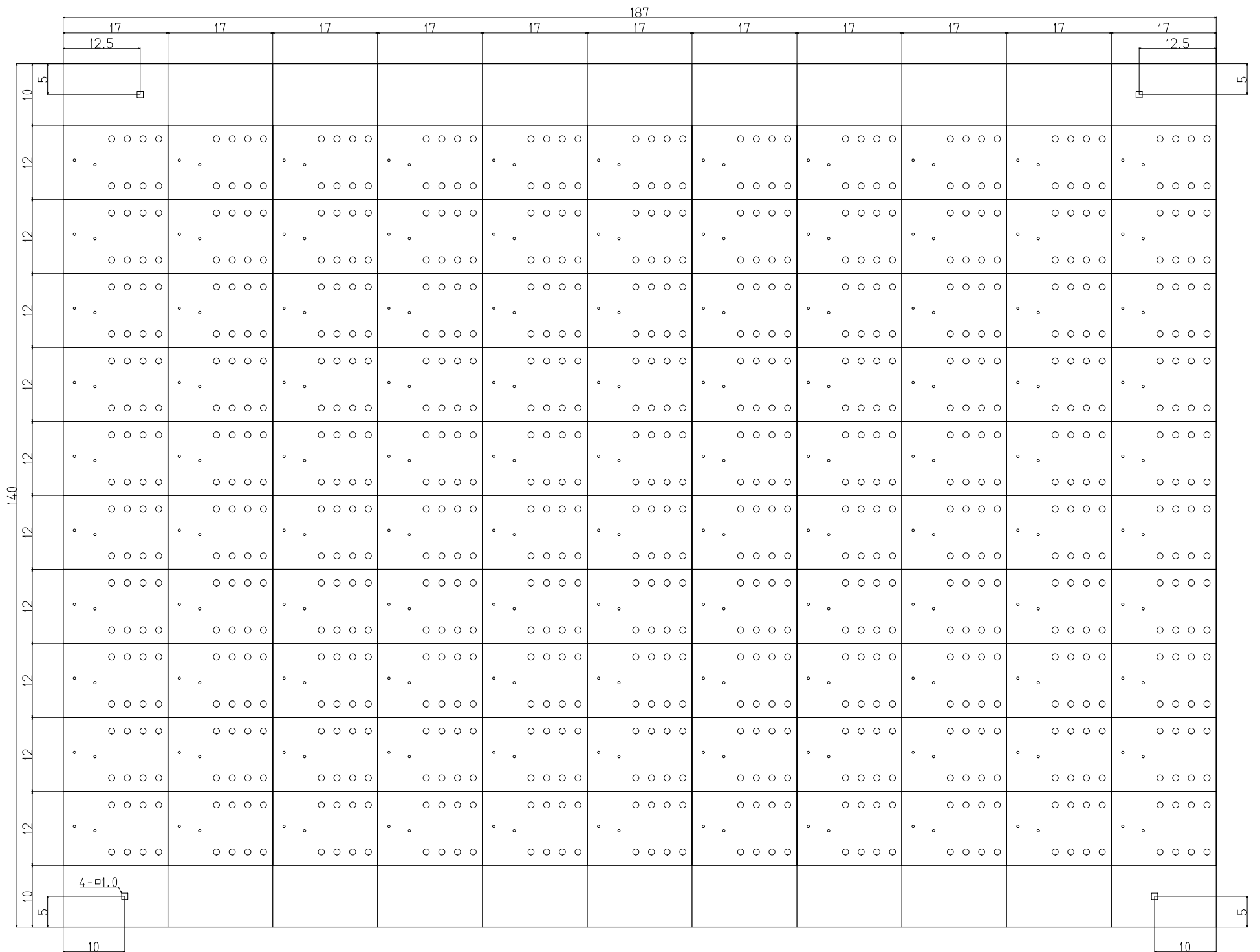
AE-1. 27X8P 集合外形图
