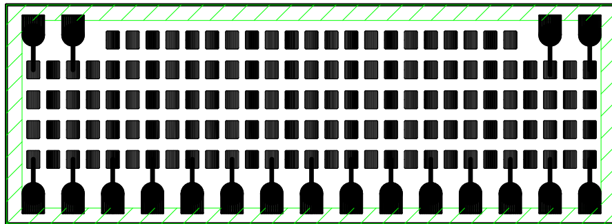
BOT (半田面パターン)
