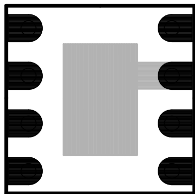
BOT (半田面パターン)
