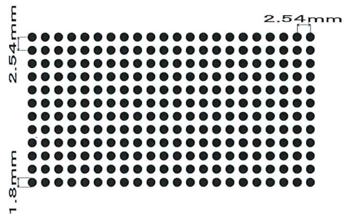
AE-FRSK120-BB-TH-I 部品面パターン (部品面視)
