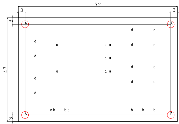
穴加工図
