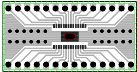
TOP (部品面パターン)
