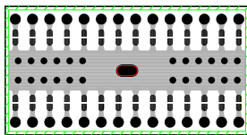
BOT (半田面パターン)
