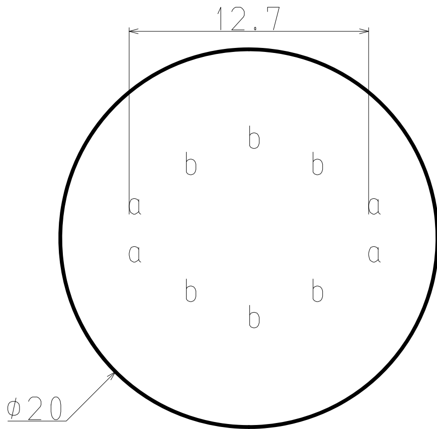
穴加工図
