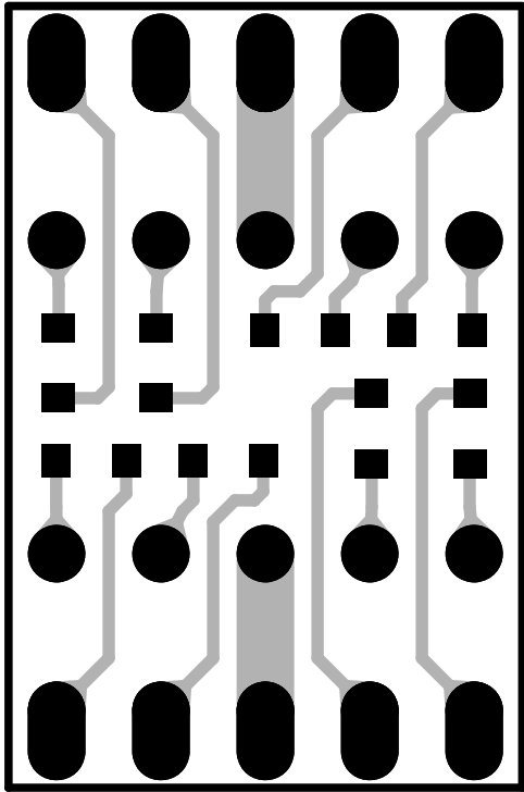
BOT (半田面パターン)
