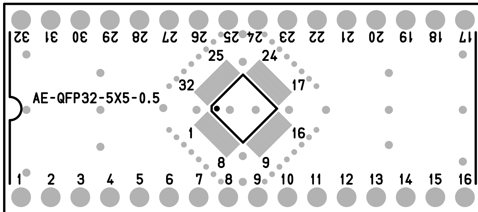
部品面シルク 部品面レジスト
