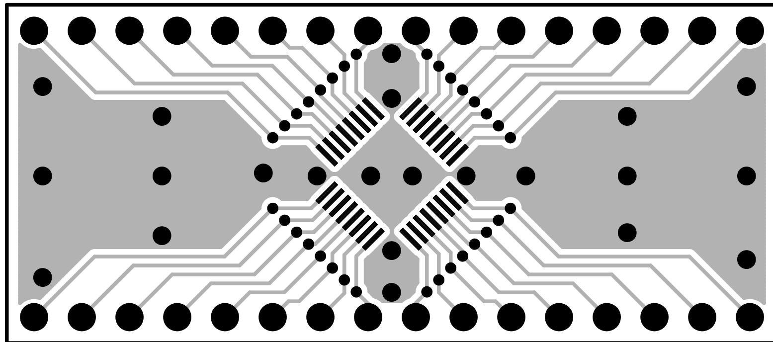
TOP (部品面パターン)
