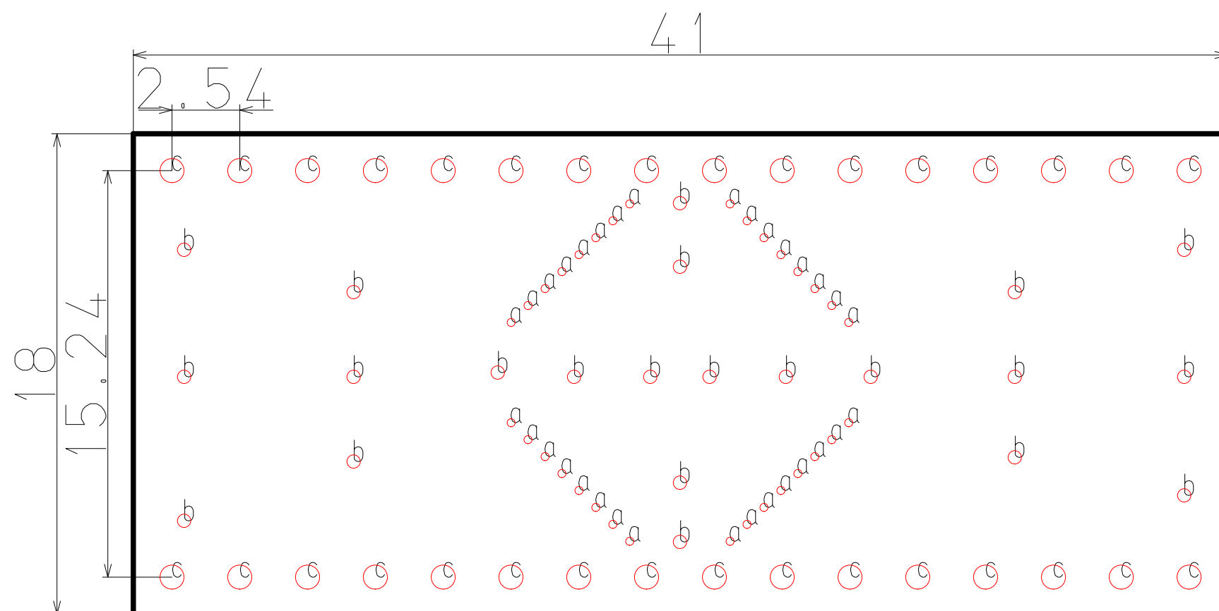
穴加工図
