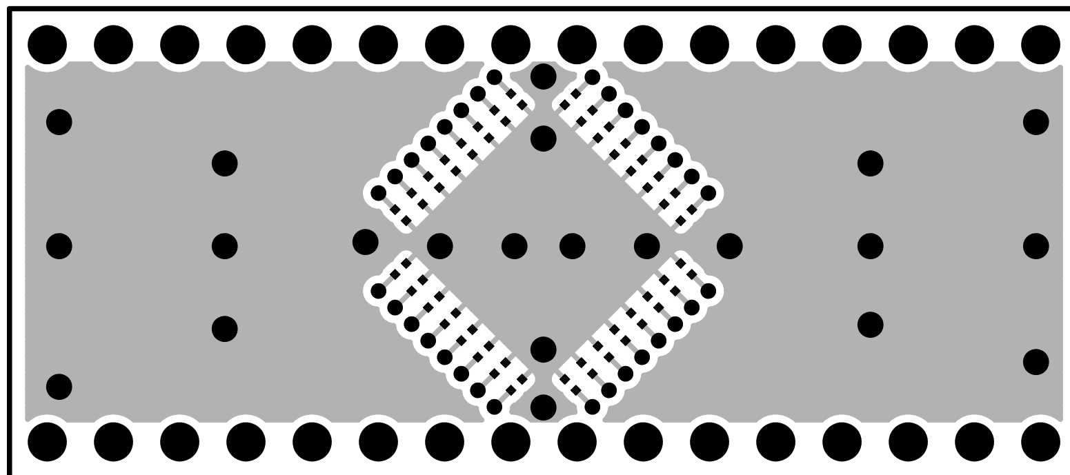
BOT (半田面パターン)
