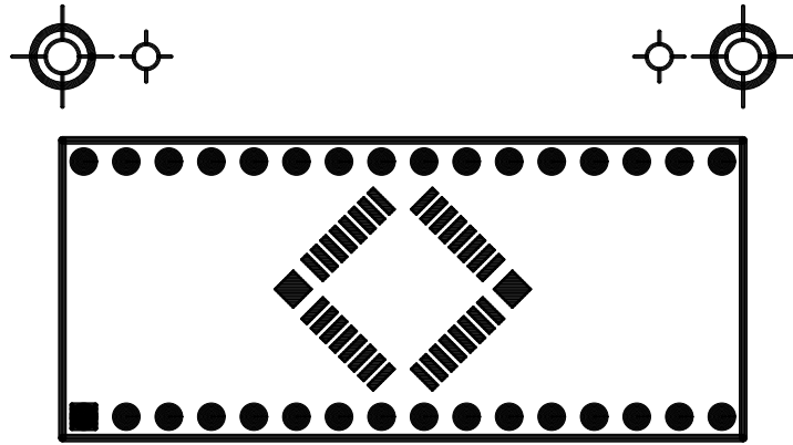
AE-QFP32-DIP 部品面レジスト
