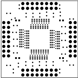
半田面レジスト
