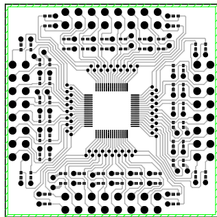
TOP (部品面パターン)
