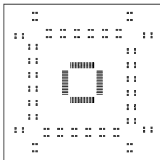
部品面メタル
