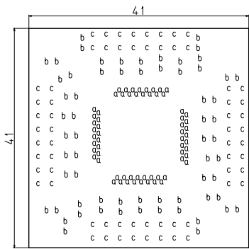
穴加工図
