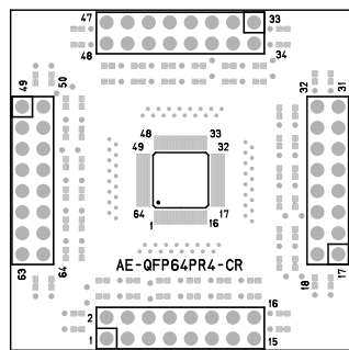
部品面シルク 部品面レスト
