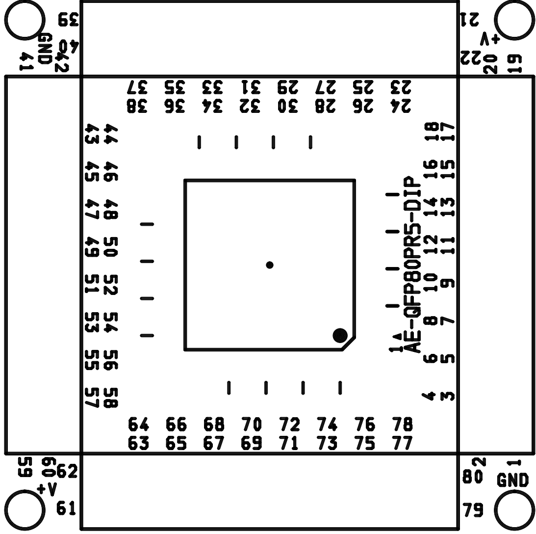
AE-QFP80PRS-DIP 部品面シルク
