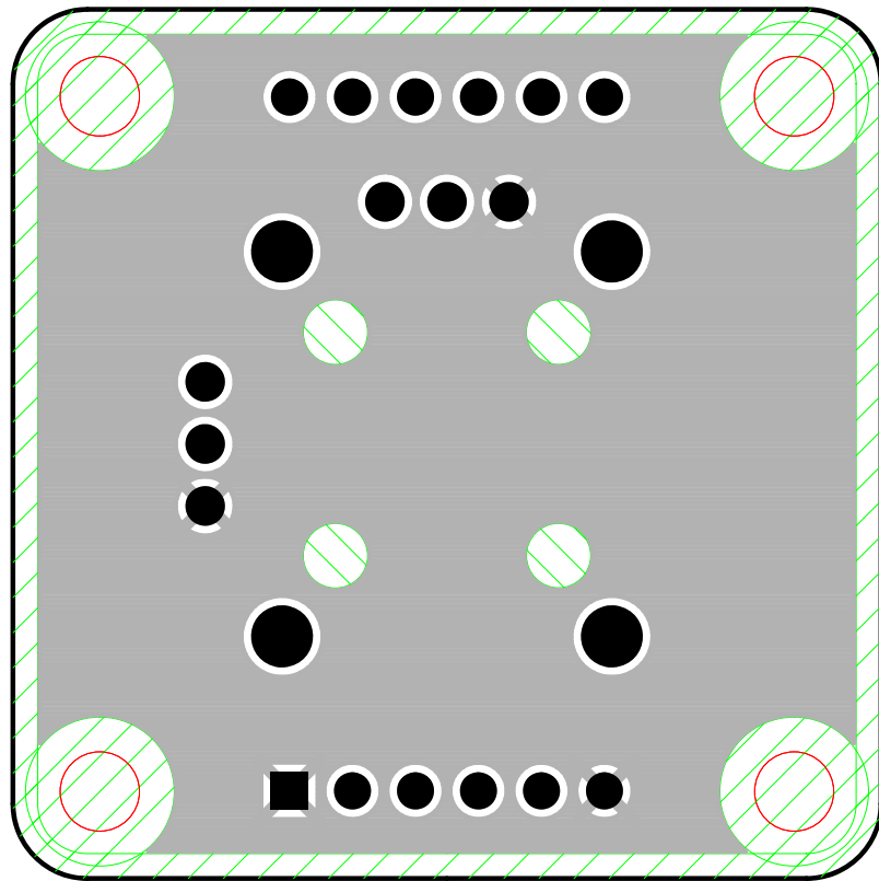
TOP (部品面パターン)
