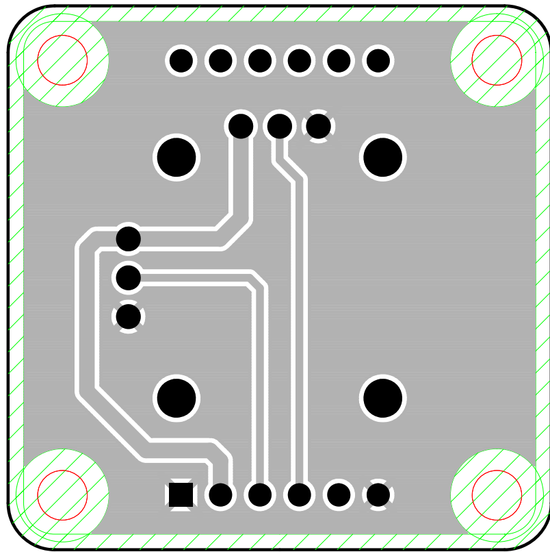
BOT (半田面パターン)
