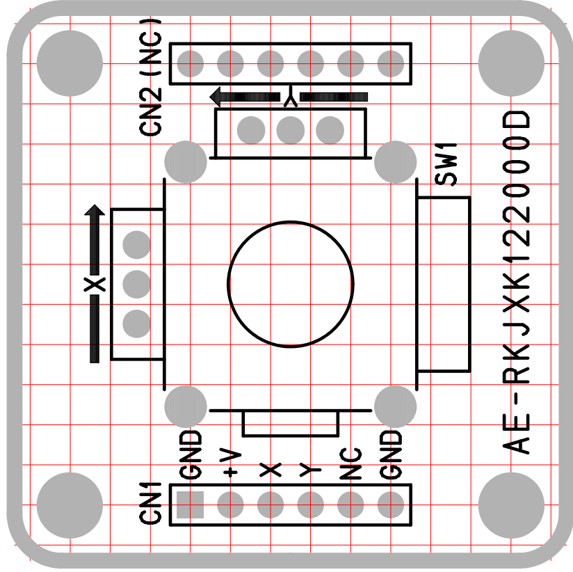
部品面シルク 部品面レジスト
