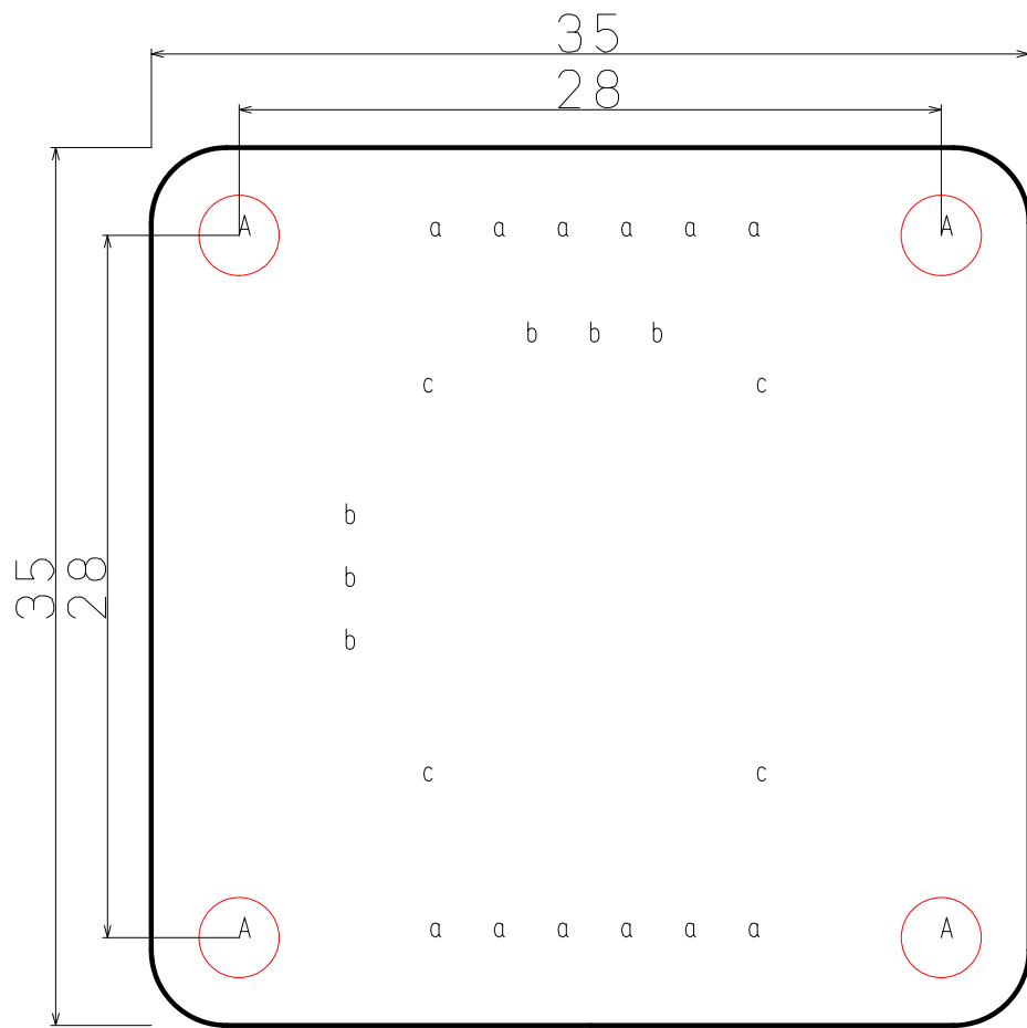
穴加工図
