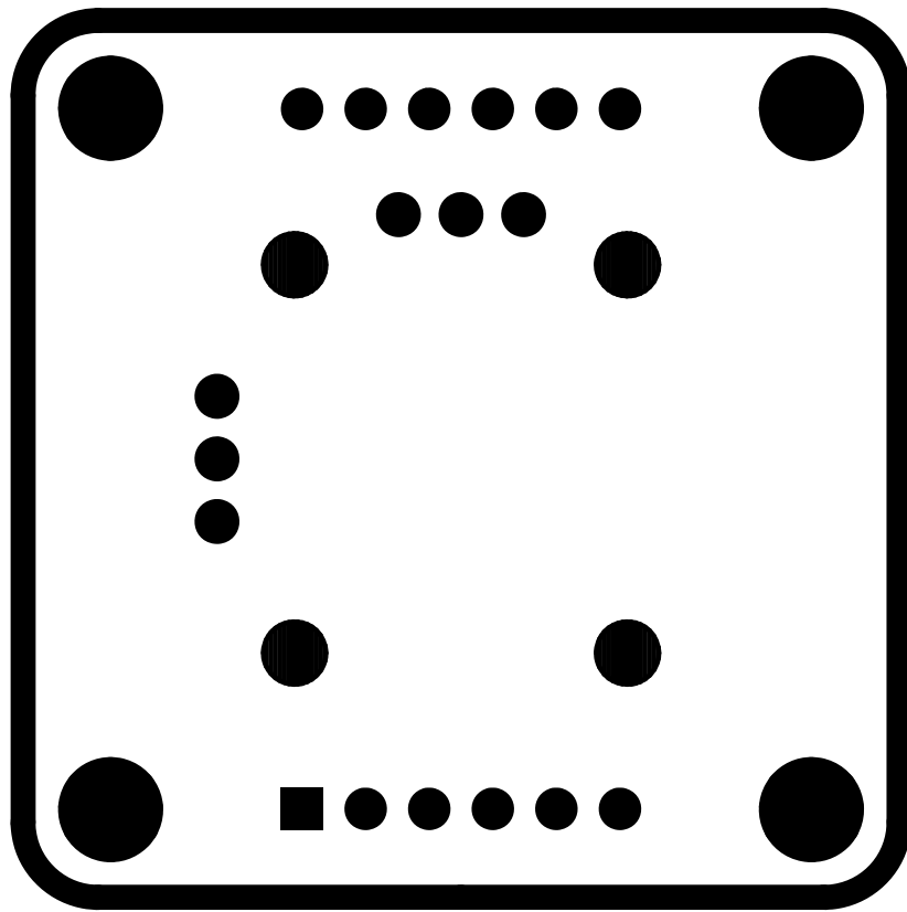
部品面レジスト
