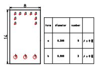
穴加工图
