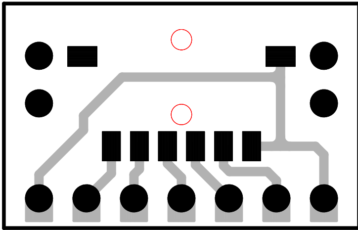
TOP (部品面パターン)
