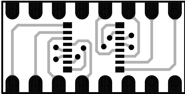
TOP (部品面パターン)
