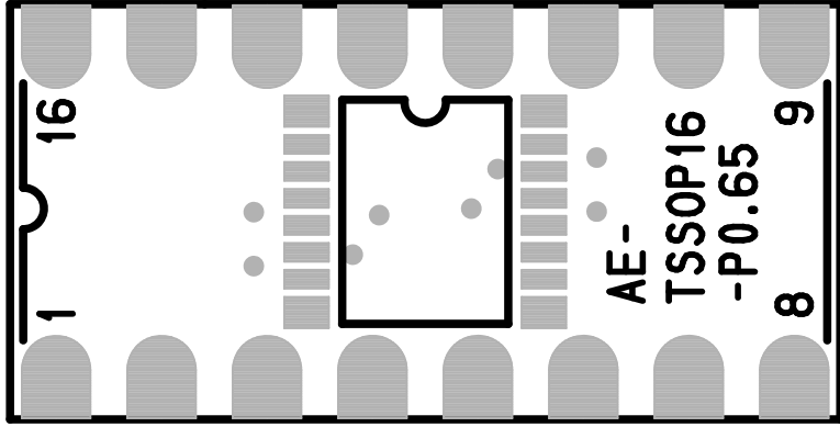
部品面シルク 部品面レジスト
