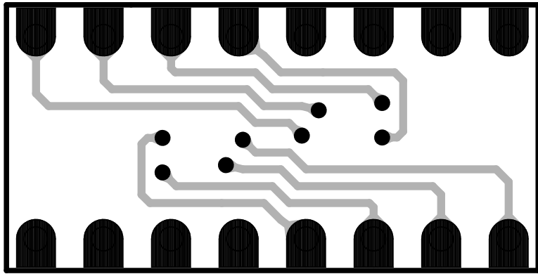
BOT (半田面パターン)
