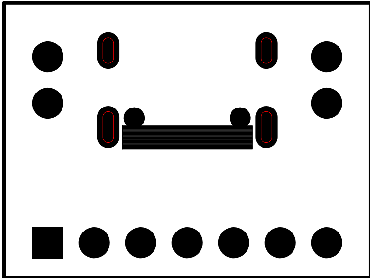
部品面レジスト
