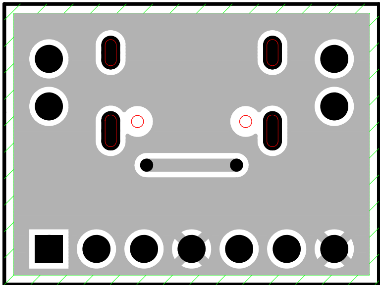
BOT (半田面パターン)
