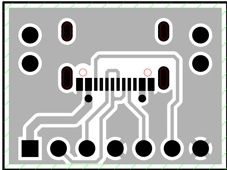
TOP (部品面パターン)
