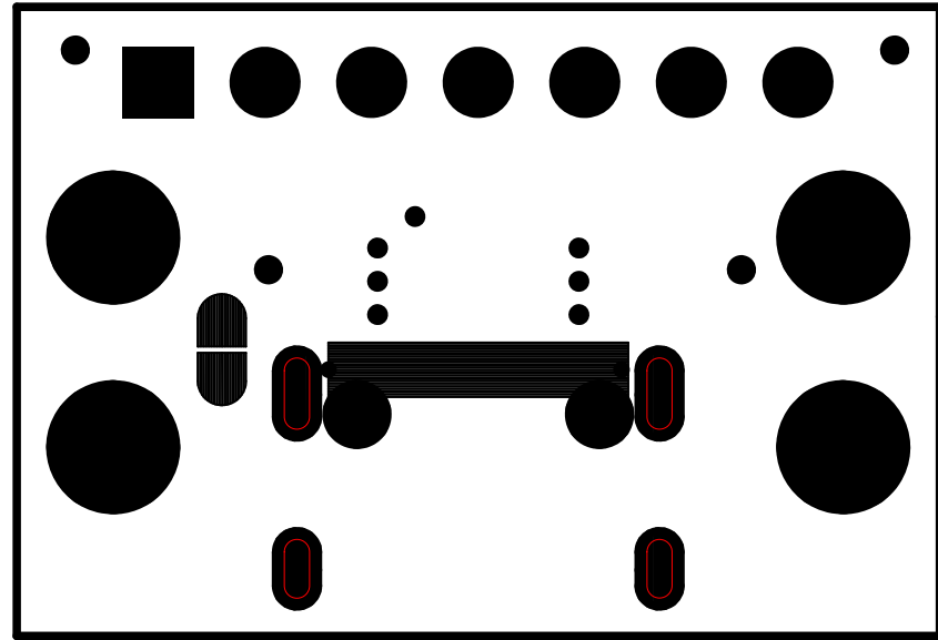
部品面レジスト
