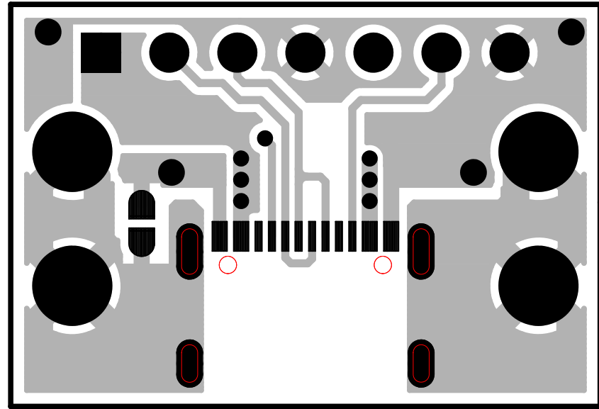
TOP (部品面パターン)
