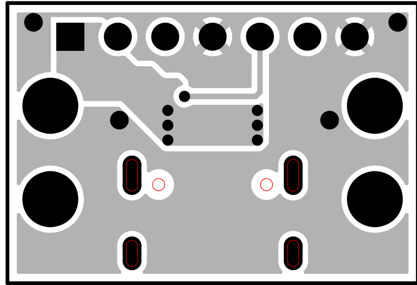
BOT (半田面パターン)
