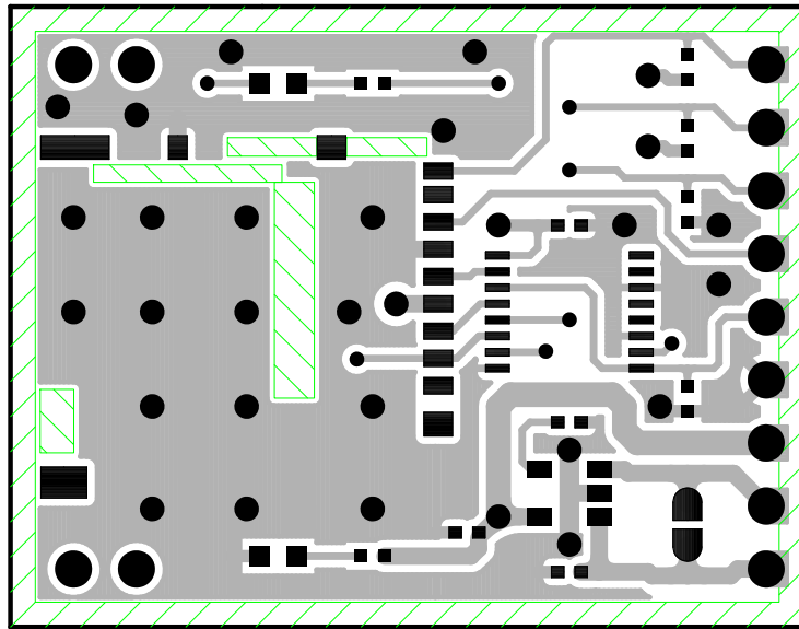
TOP (部品面パターン)
