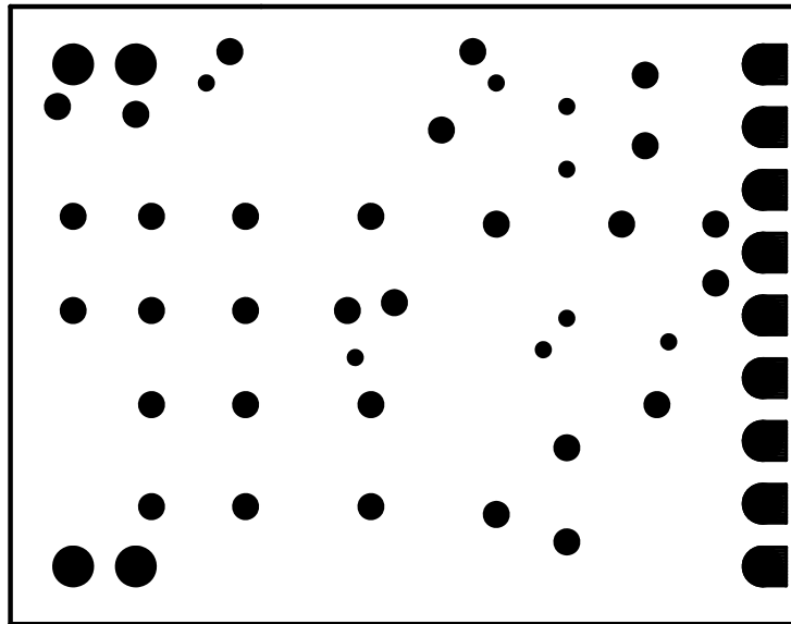
半田面レジスト
