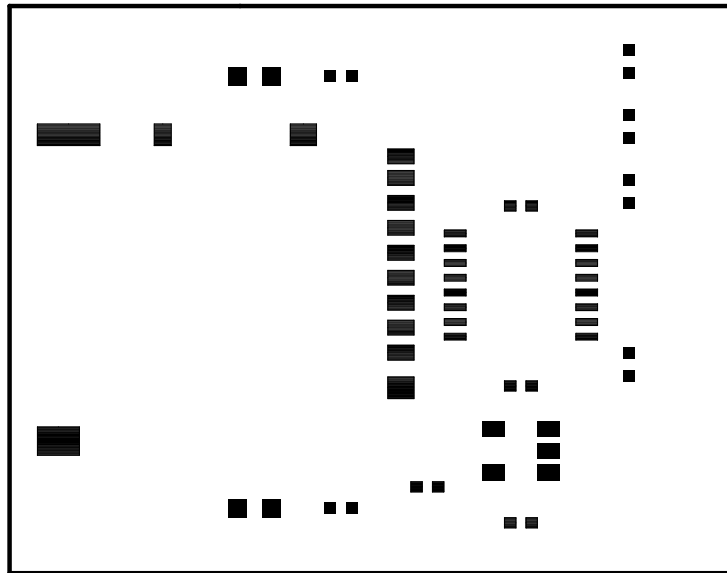
部品面メタル
