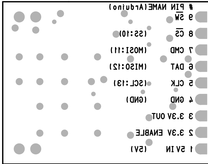
半田面シルク 半田面レジスト
