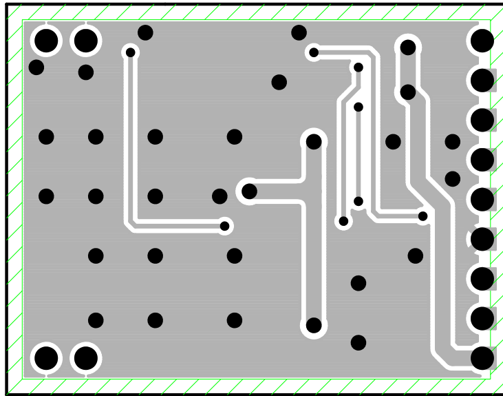
BOT (半田面パターン)
