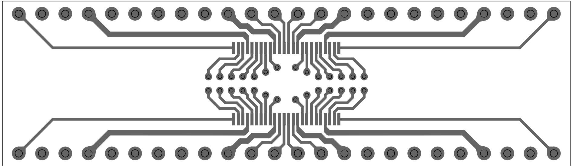
AE0.5-48P 表面パターン図
