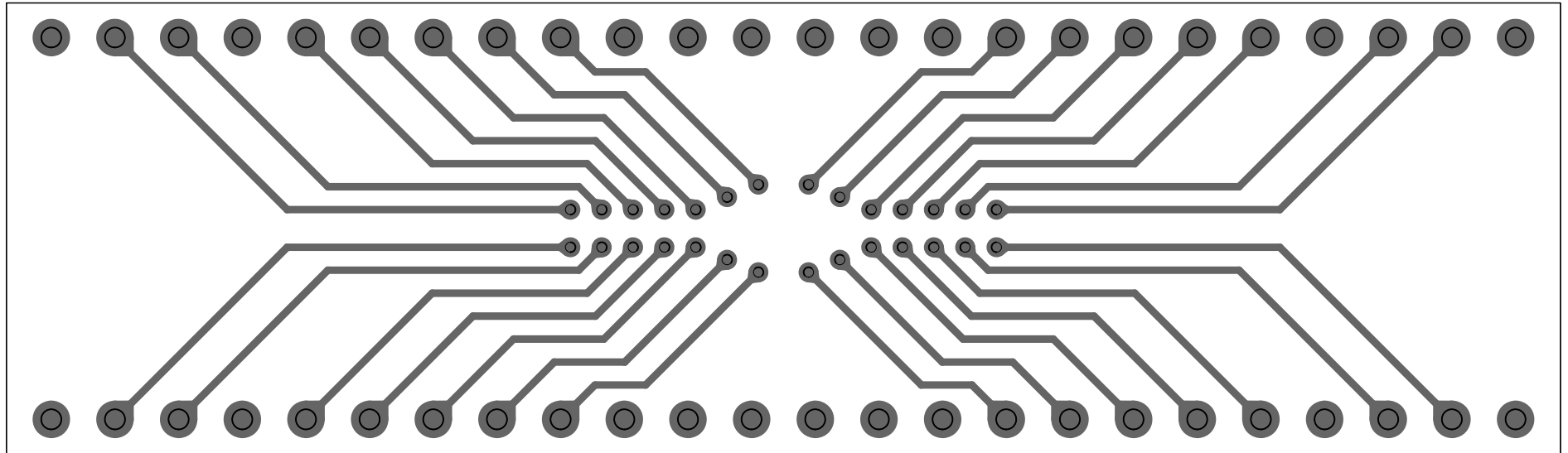
AE0.5-48P 裏面パターン図
