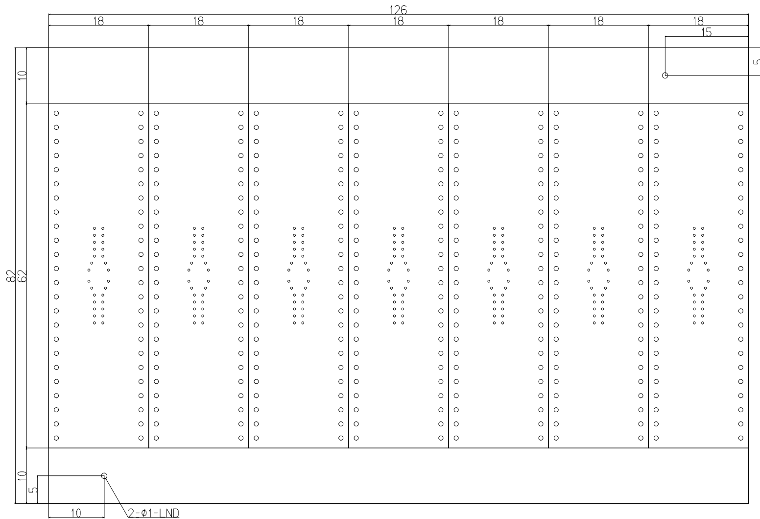
AE0.5-48P 集合外形図
