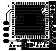
AE-ESP32-PICO-V3-ZERO TOP
