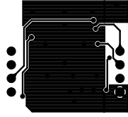
AE-ESP32-PICO-V3-ZERO BOTTOM
