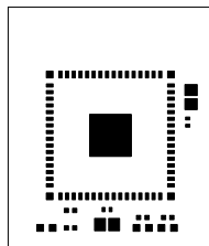
AE-ESP32-PICO-V3-ZERO TOP-METALMASK
