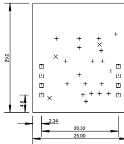
AE-ESP32-PICO-V3-ZERO
