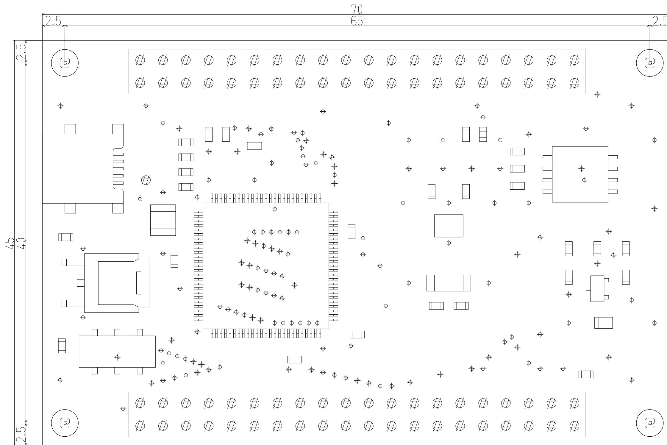
AKI-RX62 基板外形图
