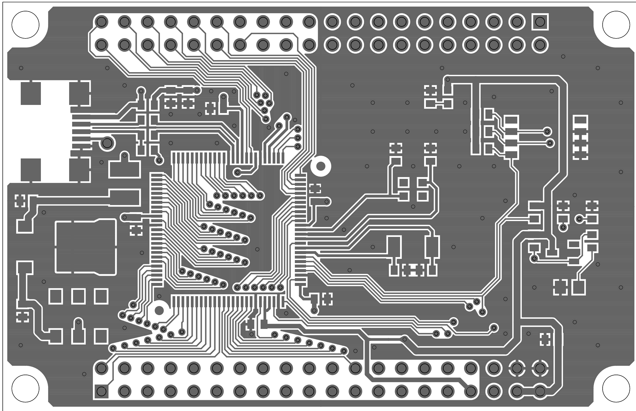
AKI-RX62 表面パターン図
