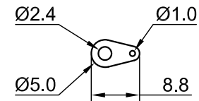
SOLDER LUG
