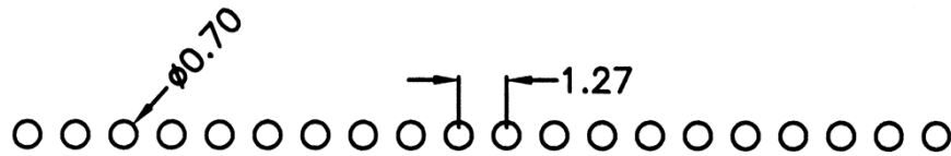
P.C.B LAYOUT
