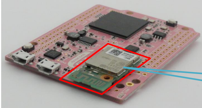
無線LANモジュール実装イメージ
