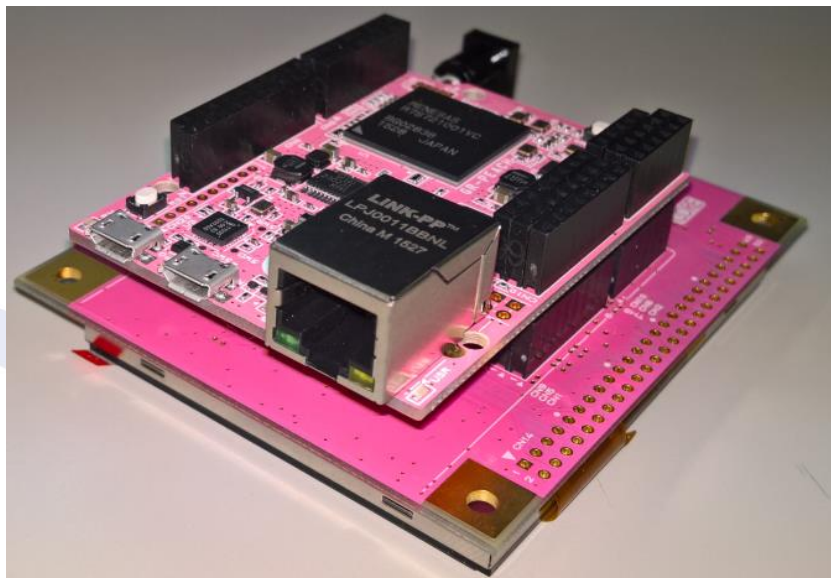
LCDシールドスタックイメージ
