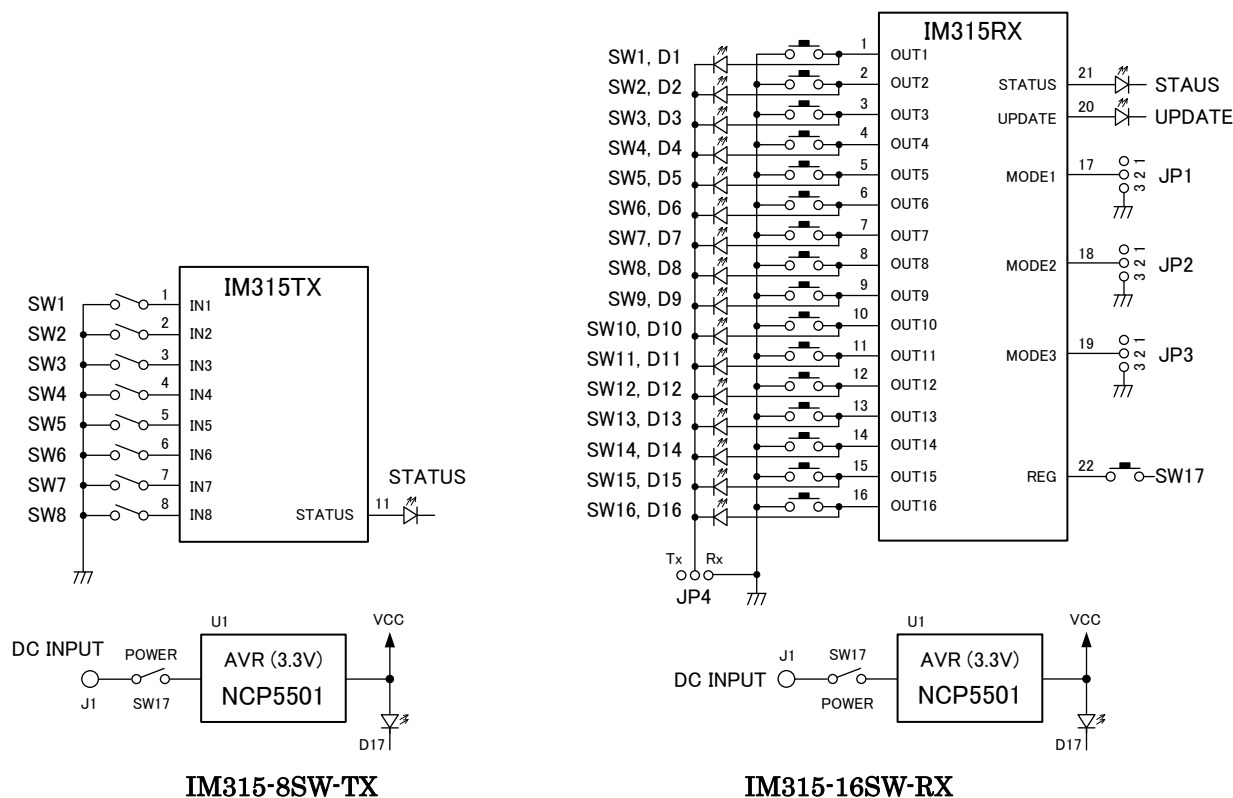
図3 ブロック図
