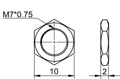
NUT
