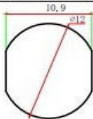
安装面板孔位推荐尺寸
