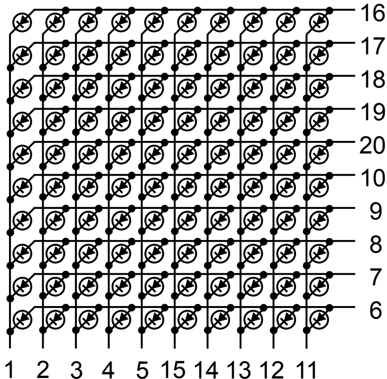
【配線図】
