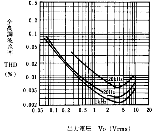
歪率対出力電圧特性例
