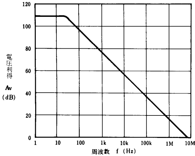
電圧利得周波数特性例
