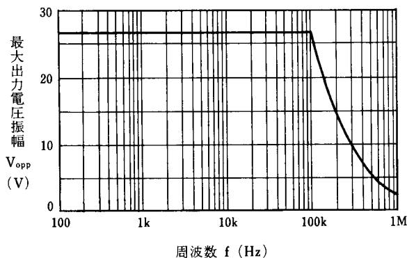
最大出力電圧振幅周波数特性例
