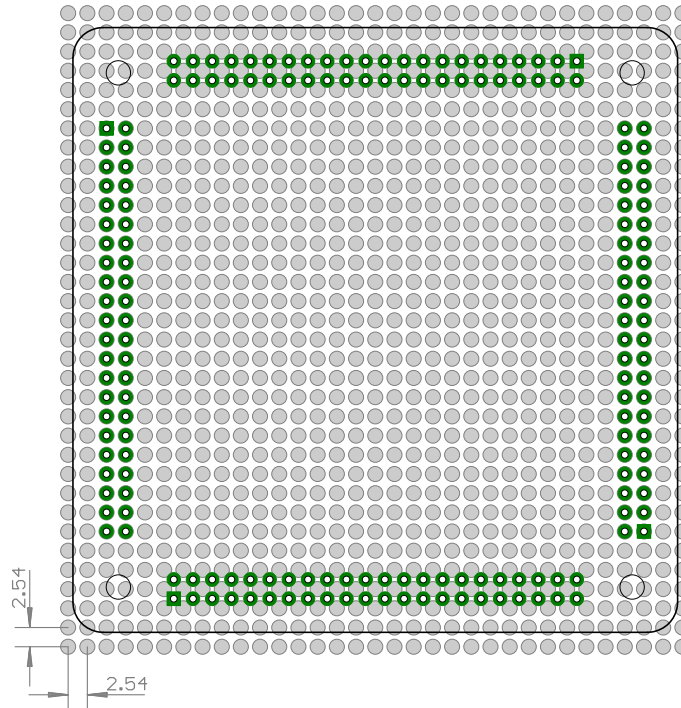
2.54mmグリッド
