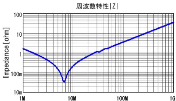
■RDE5C1H104J2K1H03B |Z| DC0V, 25degC
