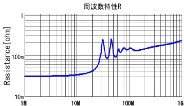
■RDE5C1H104J2K1H03B R DC0V, 25degC
