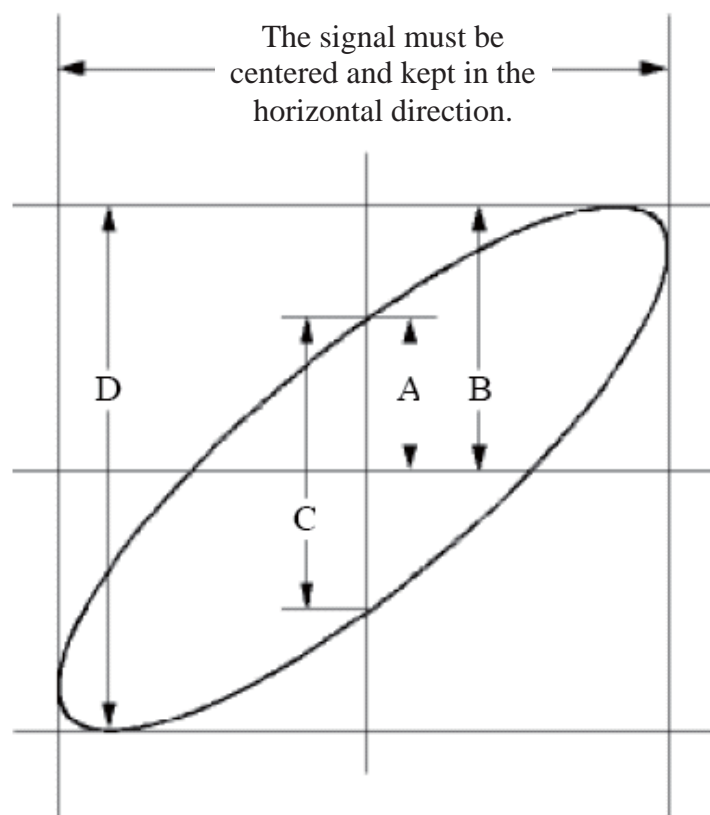
Fig.6-6 Lissajous Graph
