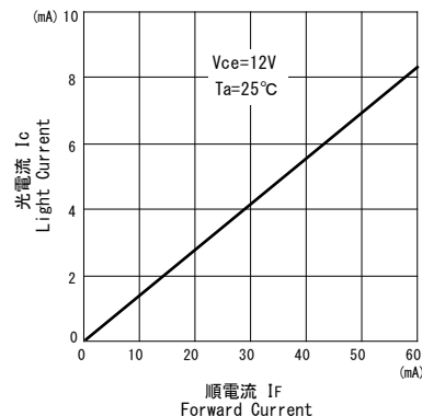
■ 光電流/順電流特性 I_c/I_F
