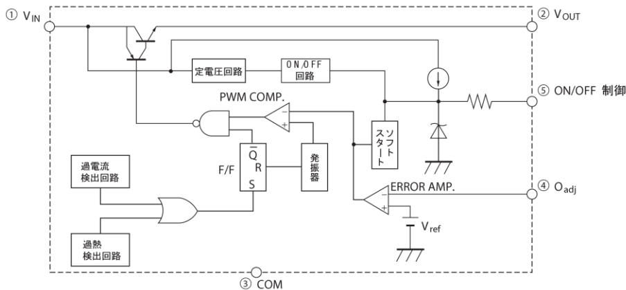
ブロック図
