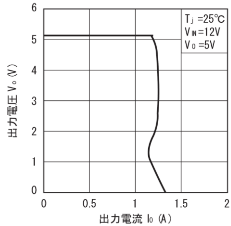
過電流保護特性 (代表値)
