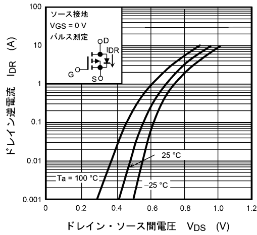
図 8.9 I_{DR} - V_{DS}
