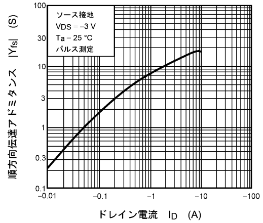
図 8.8 |Y_{fs}| - I_D
