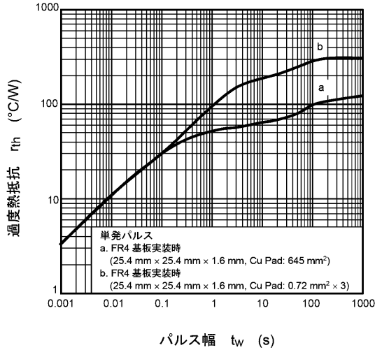
図 8.13 r_{th} - t_w
