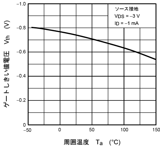
図 8.7 V_{th} - T_a
