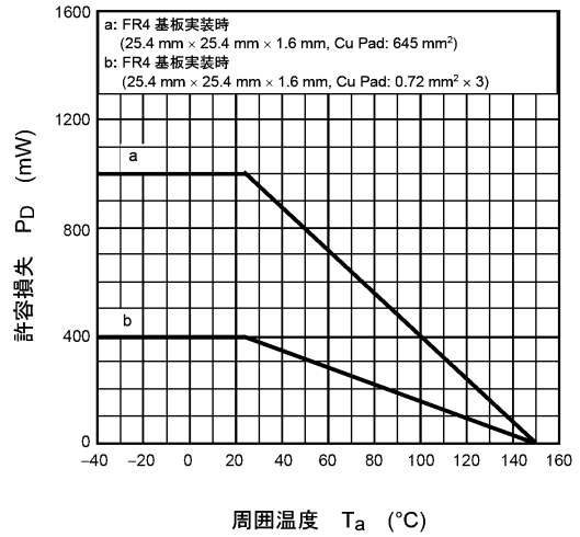
図 8.14 P_D - T_a
