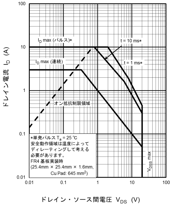
図 7.13 安全動作領域
