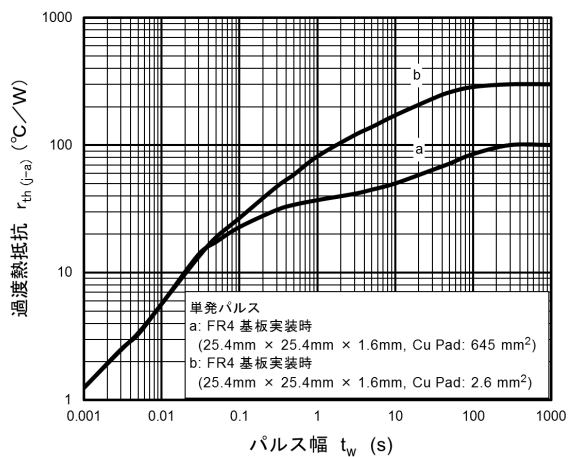
図 7.13 r_{th} - t_w
