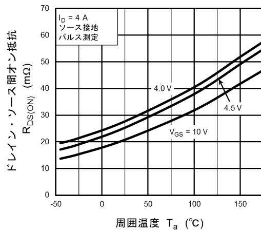
図 7.6 R_{DS(ON)} - T_a
