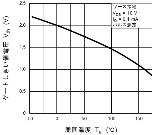
図 7.7 V_{th} - T_a
