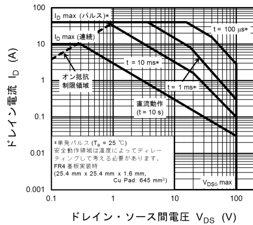
図 7.12 安全動作領域
