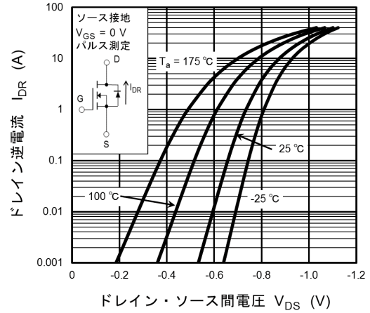
図 7.8 I_{DR} - V_{DS}
