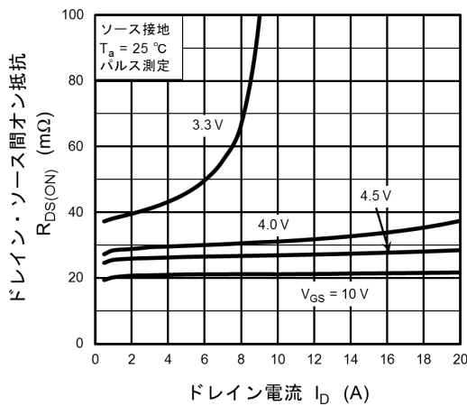
図 7.5 R_{DS(ON)} - I_D
