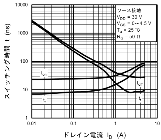
図 7.10 t - I_D
