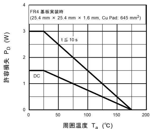
図 7.14 P_D - T_a
