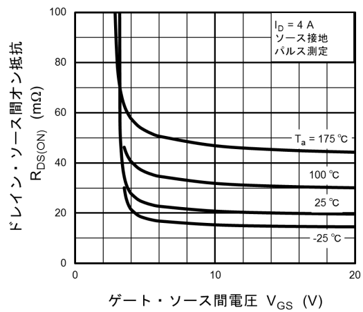
図 7.4 R_{DS(ON)} - V_{GS}
