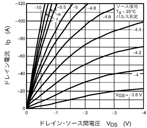
図 8.2 I_D - V_{DS}
