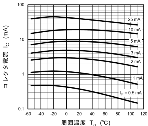
図 11.13 I_C - T_a
