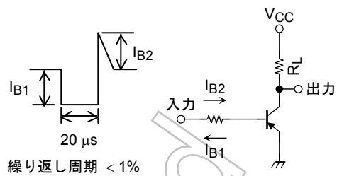
図 2. スイッチング時間測定回路 (PNP)
