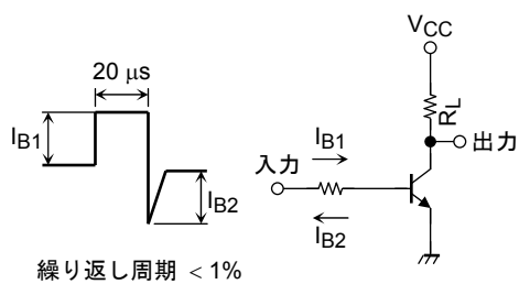
図 1. スイッチング時間測定回路 (NPN)
