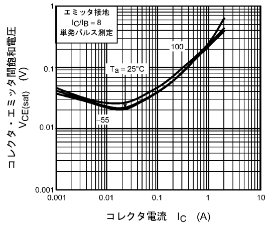
図 7.4 V_{CE(sat)} - I_c
