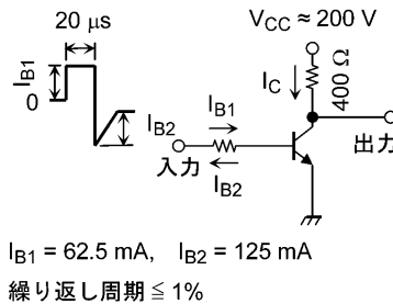
図 5.2.1 スwitching時間の測定回路
