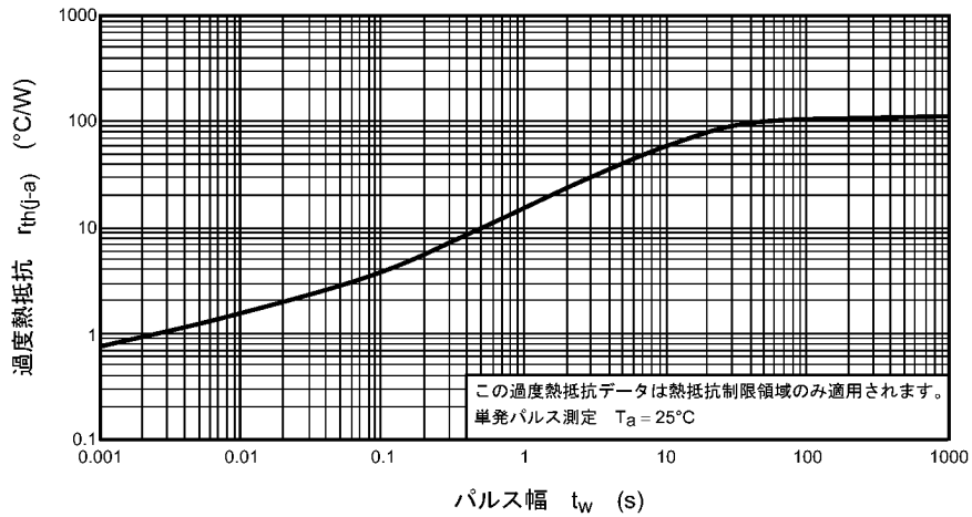
パルス幅 t_w (s) 図 7.7 r_{th(j-a)} - t_w (最大値 (保証値))
