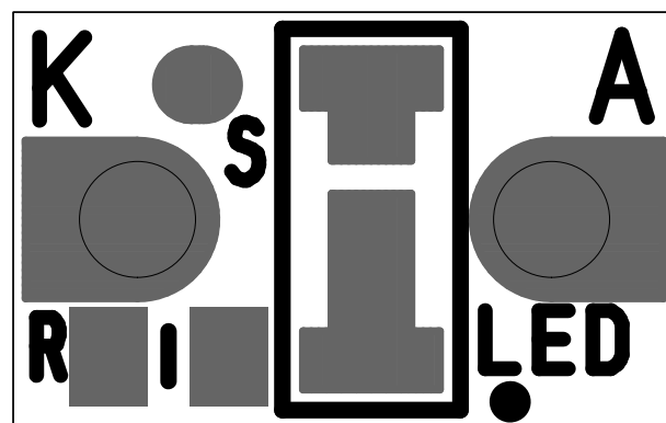
AE-LED-DIP 表面レジスト・シルク図
