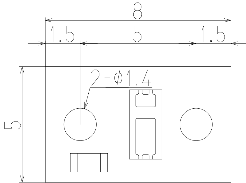
AE-LED-DIP 基板外形图
