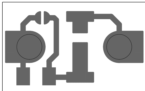
AE-LED-DIP 表面パターン図
