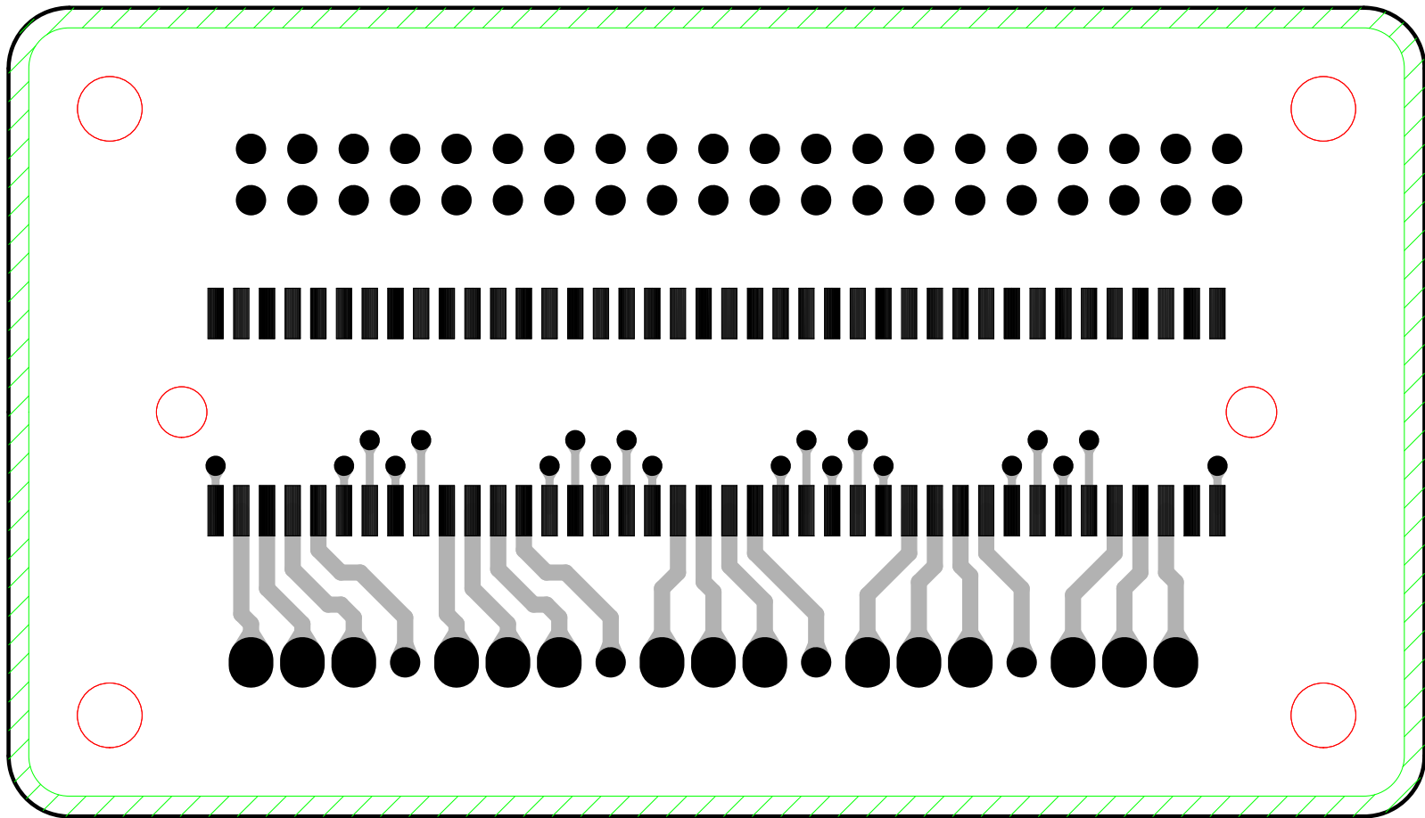
TOP (部品面パターン)
