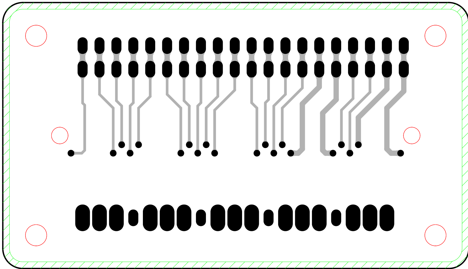
BOT (半田面パターン)
