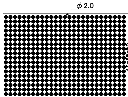
AE-SB-DIP-WD L1-PATTERN
